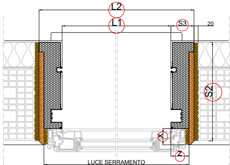
Sezione Orizzontale
