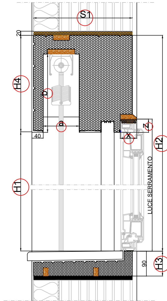
Sezione Verticale
