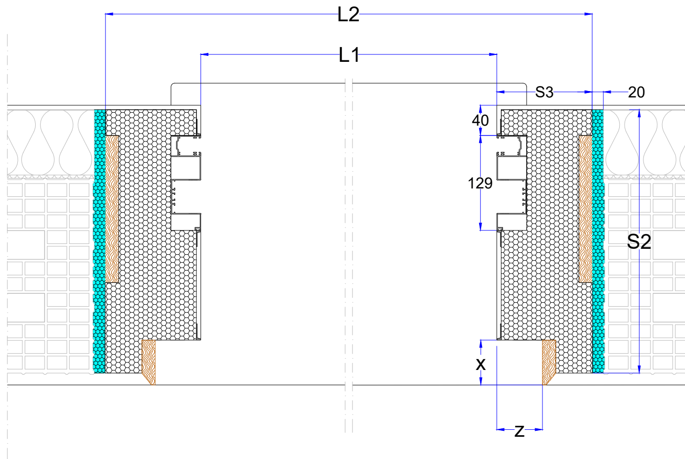
S e z i o n e O r i z z o n t a l e
