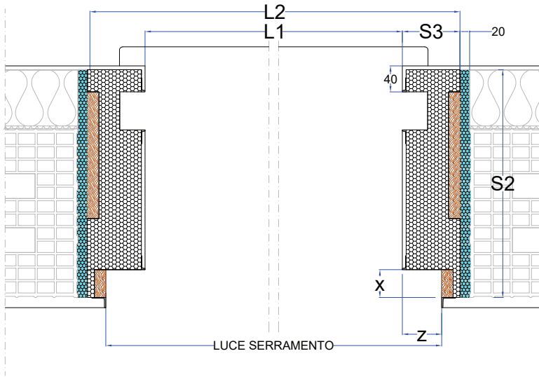
Sezione Orizzontale
