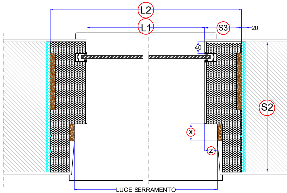
Sezione Orizzontale
