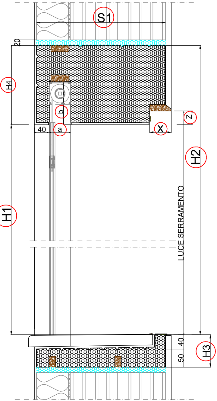
S e z i o n e V e r t i c a l e
