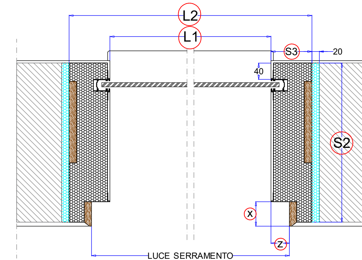
Sezione Orizzontale
