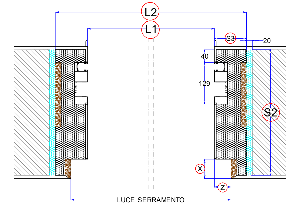
Sezione Orizzontale
